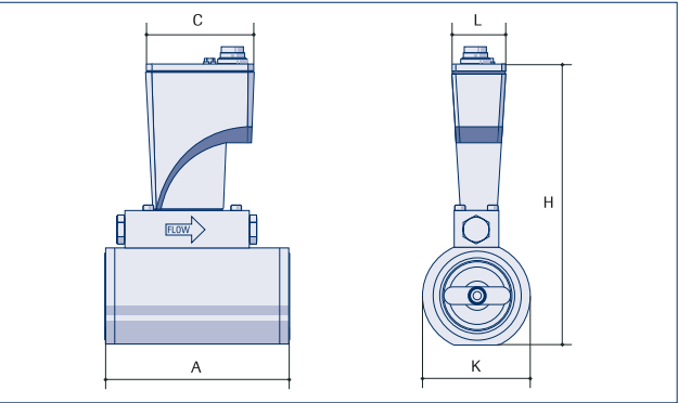
Расходомер в корпусе IP65 на большие расходы, меж-фланцевое соединение
