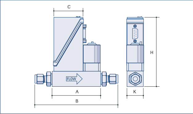
Регулятор расхода в корпусе IP40
