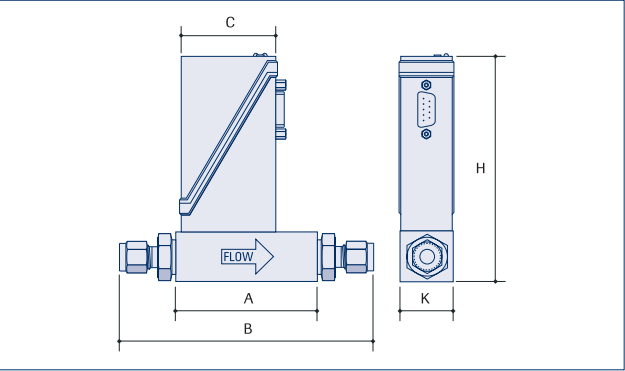
Расходомер в корпусе IP40
