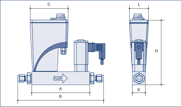
Регулятор расхода в корпусе IP65
